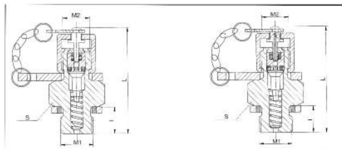
不带排气的测压接头
