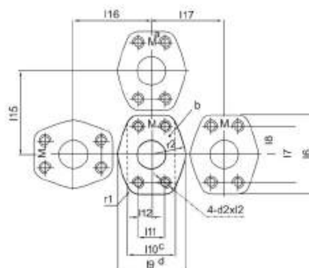
a 公制螺纹油口标记 Metric Thread Port Mark c 法兰衬垫最小宽度 Flange Washer Min. Width
