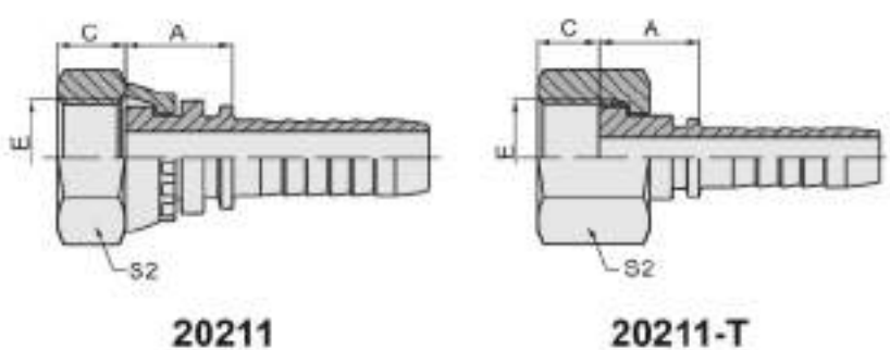
公制内螺纹平面 METRIC FEMALE FLAT SEAT 参考REF. GB/T 9065.3
