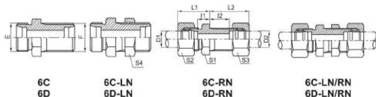
直通过板接头 STRAIGHT BULKHEAD FITTINGS
