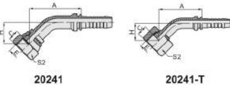
45° 公制内螺纹平面 45° METRIC FEMALE FLAT SEAT 参考REF. GB/T 9065.3
